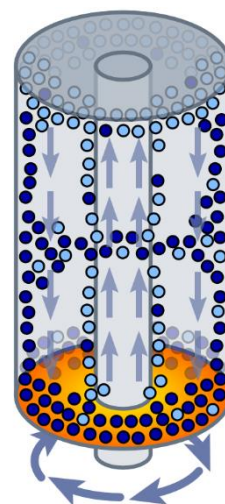
تصویر 6: سنتریفوژی که گاز در آن حرارت داده می شود: در این سنتریفوژ گاز یورانیوم هکزافلوراید از پائین داخل می گردد.
