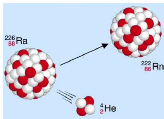
تصویر 2: از هسته رادیوم ^{226} اشعه الفا یا ذره بیرون می جهد و خودش به هسته گاز رادون ^{222} تبدیل می شود [1].
